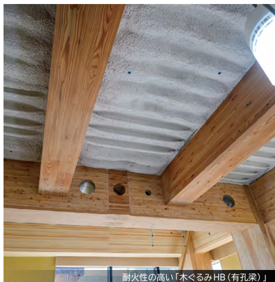
耐火性の高い「木ぐるみHB(有孔梁)」
