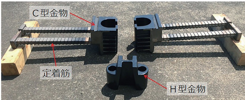
コッター継手
