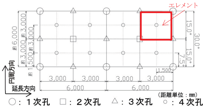
Fig. 13 孔配置展開図
