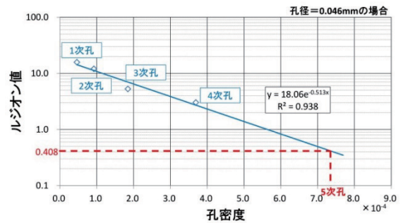
Fig. 18 ルジオン値次数通減図 (孔密度)
