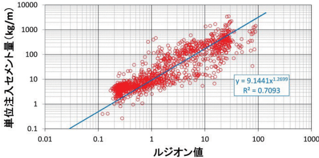
Fig. 15 ルジオン値と単位注入セメント量の関係 (規定孔全孔)
