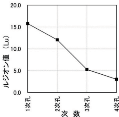
Fig. 16 ルジオン値次数通減図
