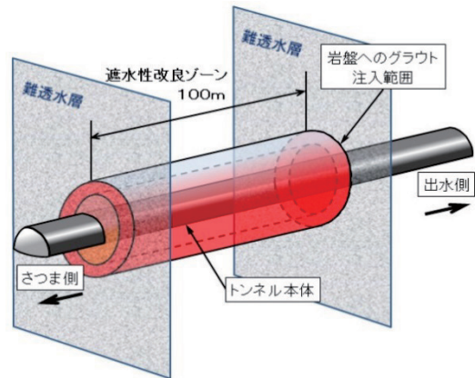
Fig. 3 減水対策工の概要図
