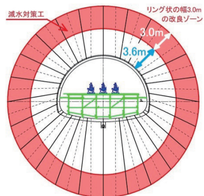
Fig. 8 改良範囲とグラウチング工法の孔配置
