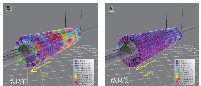
Fig. 19 改良前後のエレメント (Lu)
