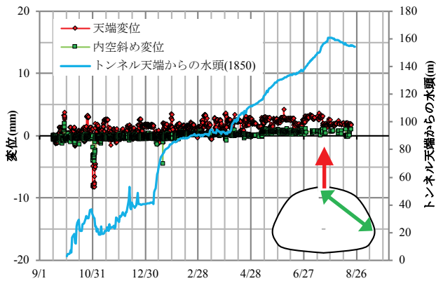
Fig. 21 トンネル内空変位と地下水位
