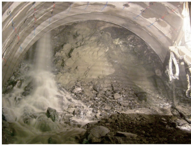
Photo. 1 貫入境界付近の掘削時の大量湧水状況
