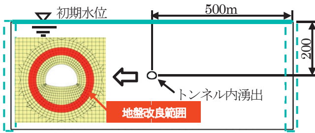
Fig. 4 浸透流解析モデル
