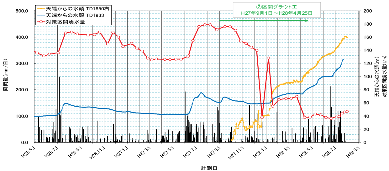
Fig. 20 対策区間湧水量とトンネル天端からの水頭の経時変化
