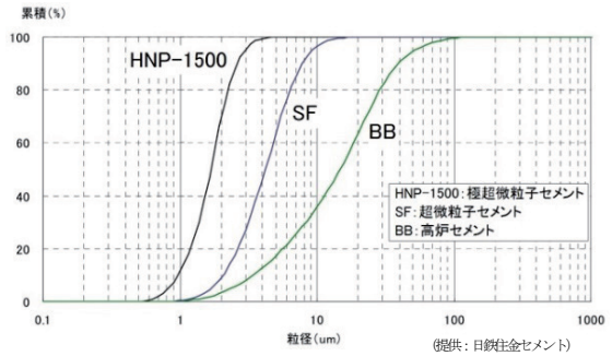
Fig. 10 各セメント粒子の粒度分布
