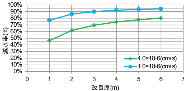
Fig. 5 改良厚および改良部透水係数と減水率
