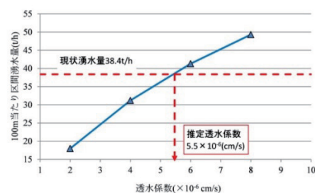
Fig. 14 浸透流解析による改良部の推定透水係数
