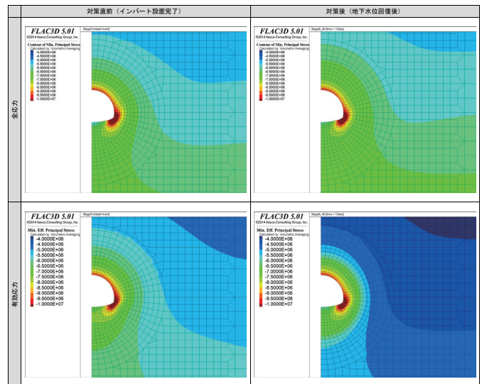
Fig. 7 トンネル周辺の応力分布
