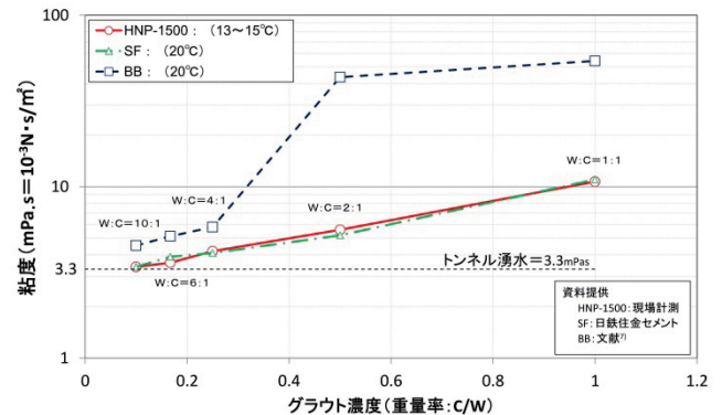
Fig. 11 グラウト材の粘度の比較
