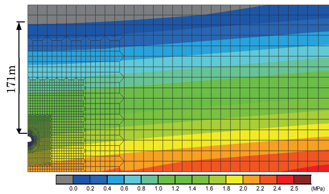
Fig. 6 減水対策後の間隙水圧分布図
