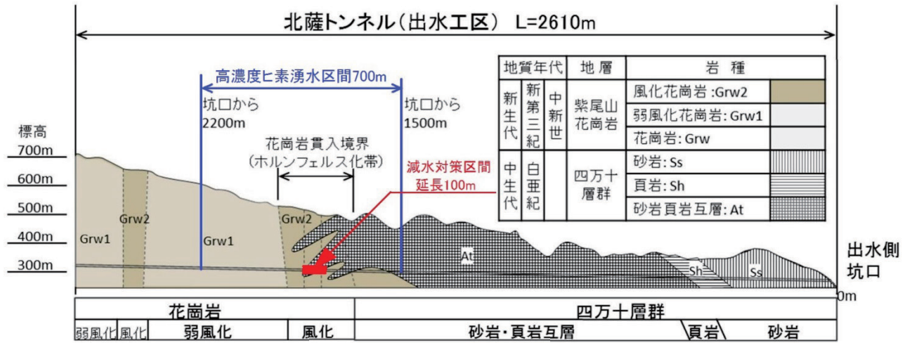
Fig. 2 地質縦断面図
