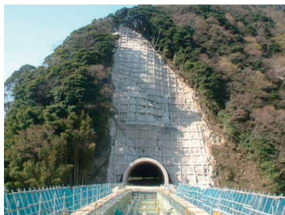
のり面对策工全景
