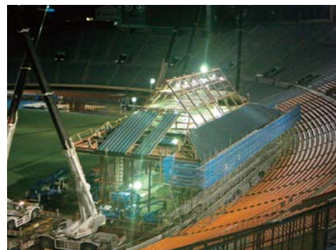
屋根パネルの施工 6月30日 22時
